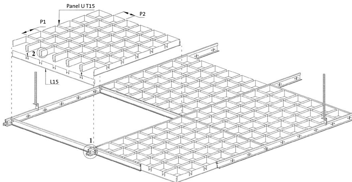
Pieza para cerrar los paneles
