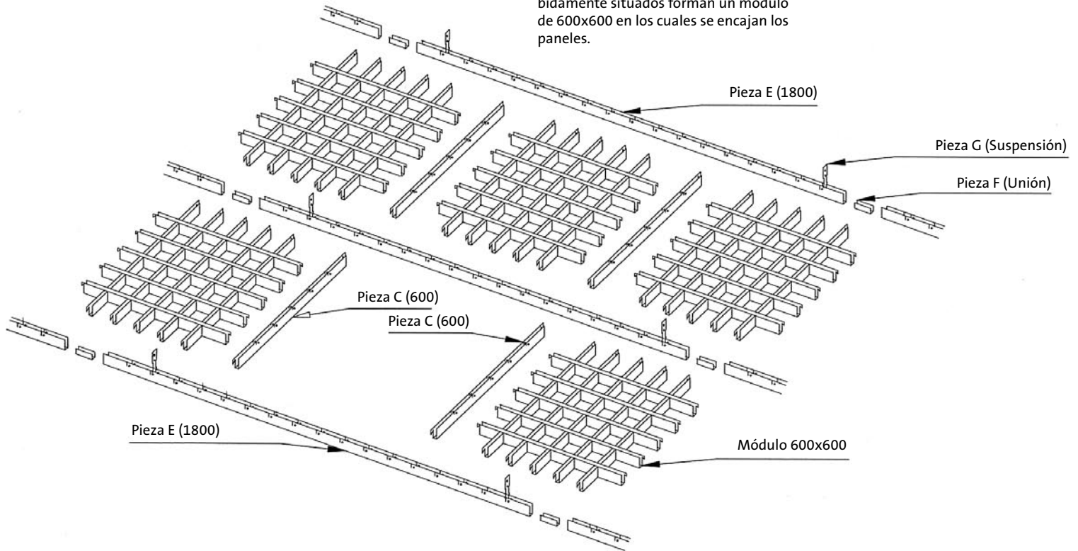
Panel de 600x600
